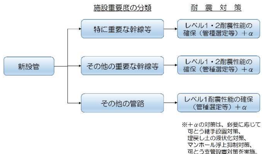
図 3.1.5 新設管の耐震対策フロー
